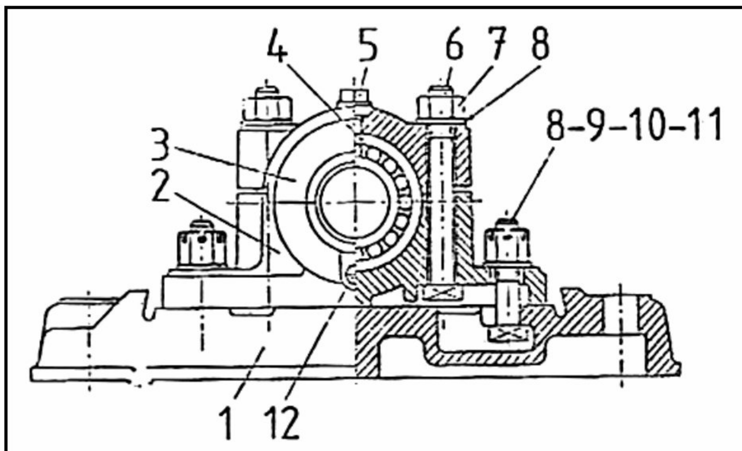
شکل ۶-۵- روش‌های معرفی اجزا
